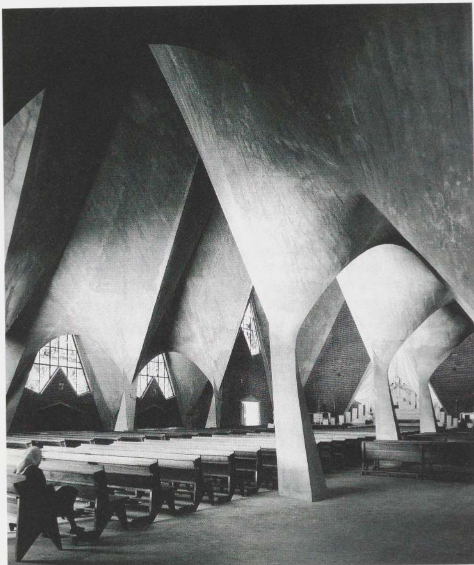
Felix Candela. Iglesia de la Virgen Milagrosa. 1954–55. Navarte, Mexico
