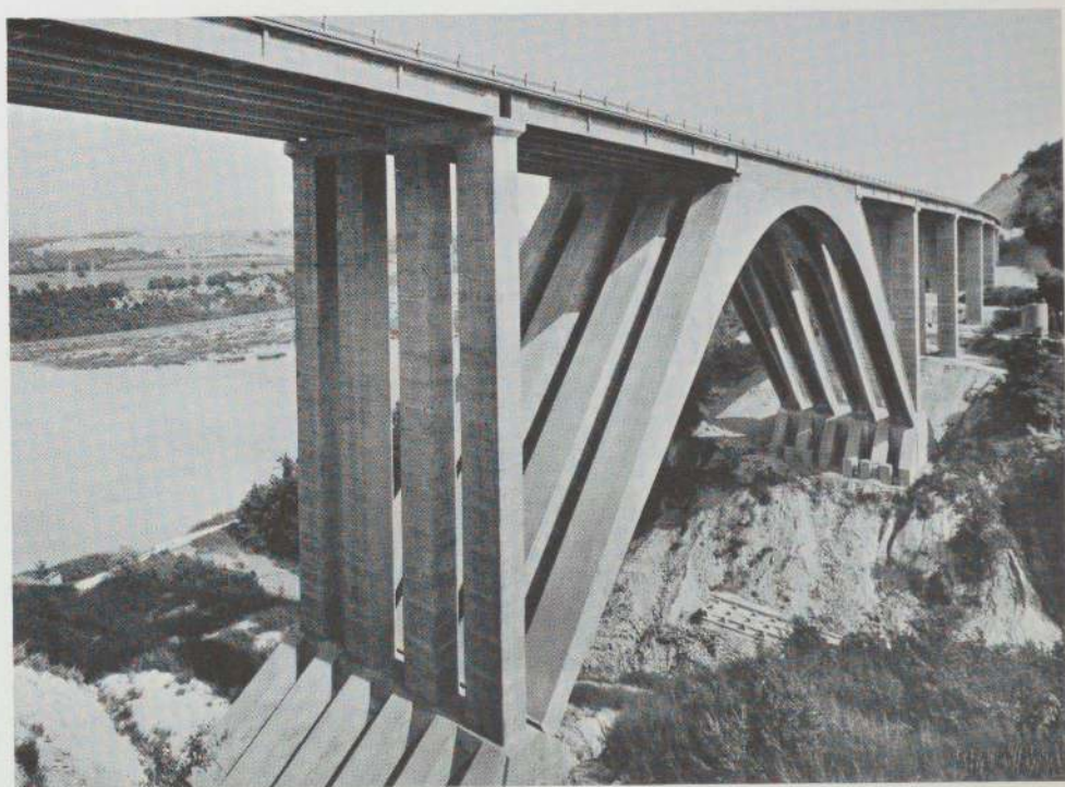
82 Poggettone and Pecora Vecchia Viaducts. Autostrada del Sole, Bologna- Florence section, Italy. 1960. Arrigo Carè, Giorgio Giannelli.
